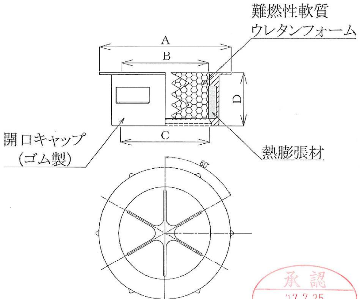
図1 断面図
