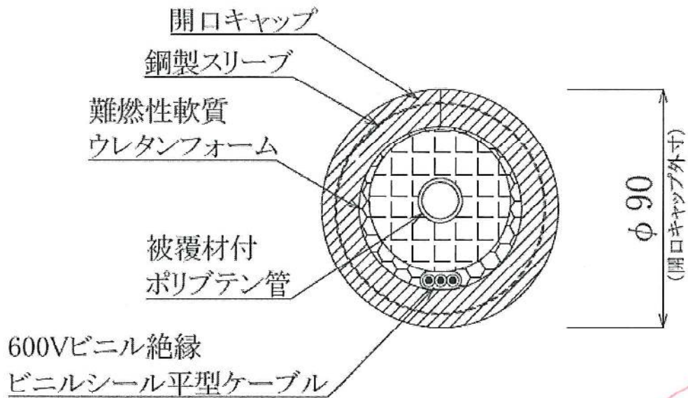
立面図
